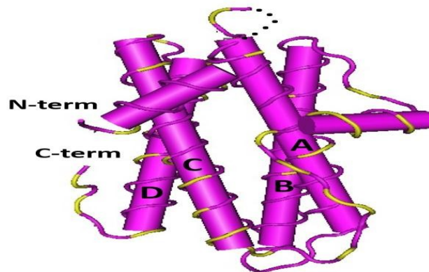
Fig.2. Alineamiento estructural de las proteínas Dpr de S. mutans y S. pyogenes . Se observan las regiones A, B, C y D, así como las porciones que corresponde a aminoácidos no conservados (amarillo).
