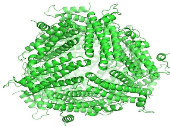
Fig. 3. Modelo tridimensional de la proteína Dpr de S. mutans . Se muestra la estructura dodecamérica de la proteína así como los posibles sitios de unión al hierro.
