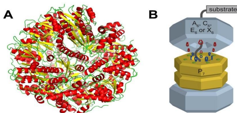
Fig. 3. (A) Modelo tridimensional de la estructura tetradecamérica de la proteasa ClpP de S. mutans . (B) Arquitectura de las proteasas-chaperonas Clp. Se destaca la ubicación de la proteasa ClpP (naranja) como parte fundamental del anillo [7].
