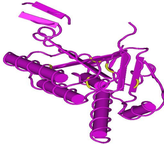
Fig. 2. Alineamiento estructural de las proteasas ClpP de S. mutans y S. pneumoniae . Se observan las porciones que corresponde a aminoácidos no conservados (amarillo).
